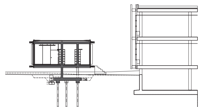
coupe transversale
