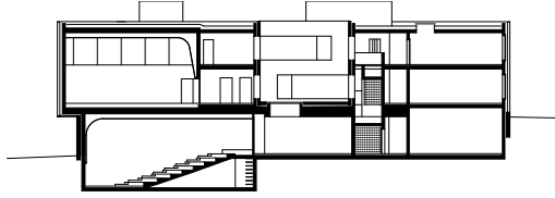
coupe longitudinale
